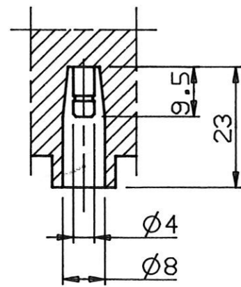
Cut A--A
