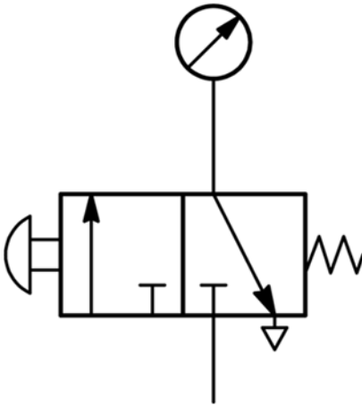
Abbildung 3: Schaltschema
